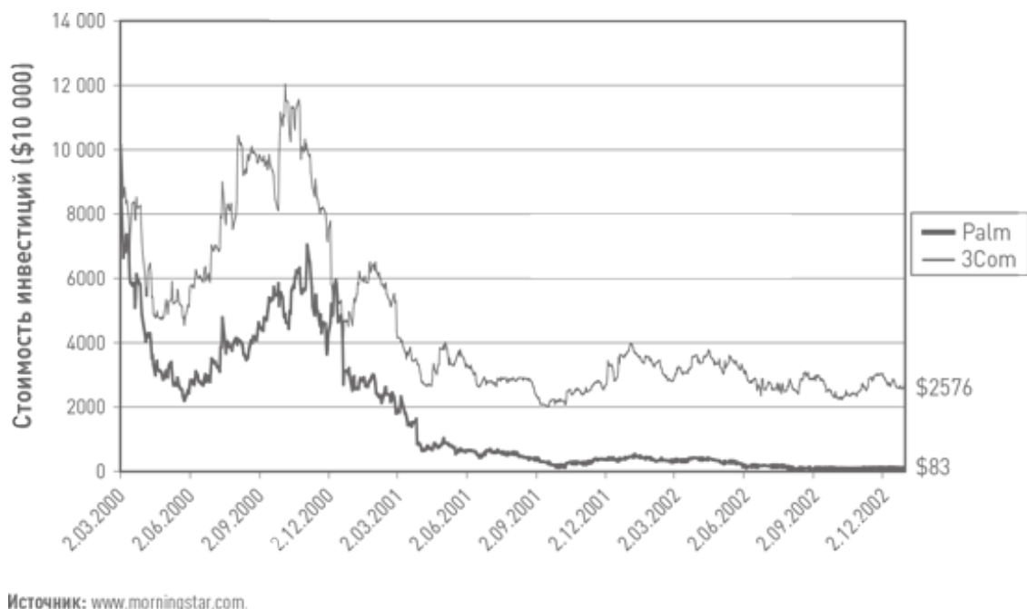
Рис. 18.1. Падение Palm
